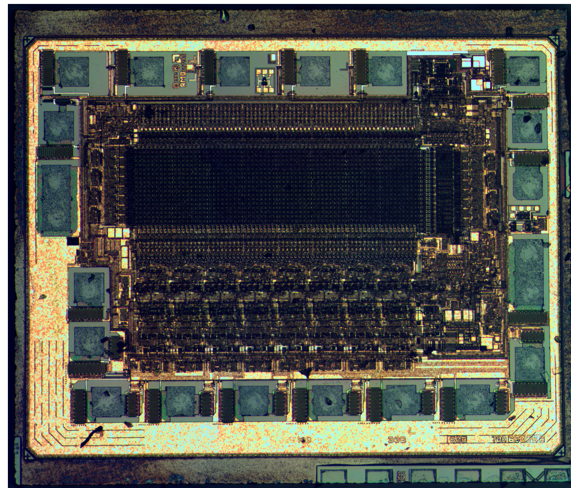
Microchip GAL(Generic array logic) vznikl jako inovace mikrochipu PAL Programmable Array Logic kolem roku 1980. velikost 2434×2079µm zdroj: https://zeptobars.com
