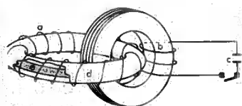
Schematische Ansicht von ZETA. a) Magnetspule zur Erzeugung eines stabilisierenden Feldes; b) Stoßtransformator zur Erzeugung des Plasmas; c) Kondensatorbatterie (gespeicherte Energie 500 000 Wattsec.); d) Ringröhre (Durchmesser 3 m); e) Plasmafaden
