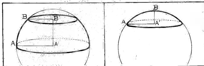
Exemples de segments sphériques.
